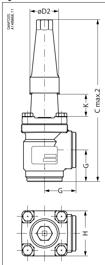
Figure 23: SVA-xx x x ANG CAP
